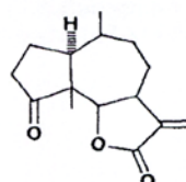
VII, Damsin
