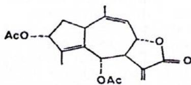
(XV)
