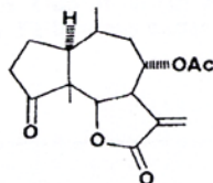
VIII, Confertiflorin
